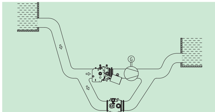
4.用于水轮机的进口启闭和旁通控制
