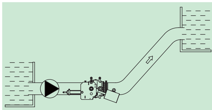
2.用于水泵出口的控制阀。开启时缓开；关闭时先快速关闭90%，然后再缓慢关闭。水头损失极小。
