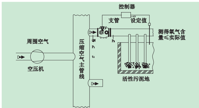
3.用作污水处理厂活性排泥池曝气管路中的空气流量控制阀
